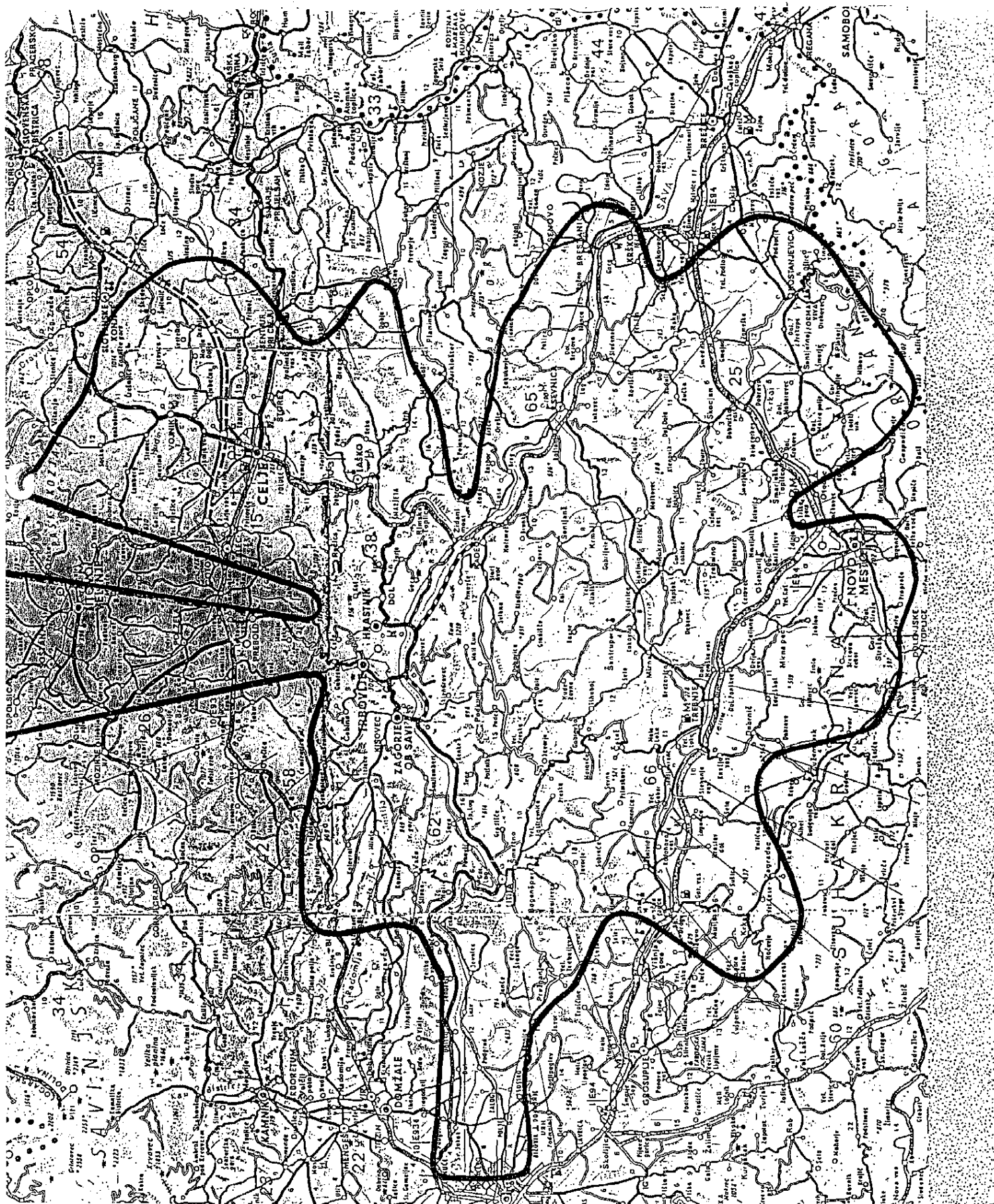
Radio Trbovlje Področje pokrivanja radijskega oddajnika Kum 98.1 Mhz, ERP = 1kW, izračunano po EBU Tech. 3236-E z uporabo CCIR krivulj. Mejna vrednost polja je 66 dBμV/m.
